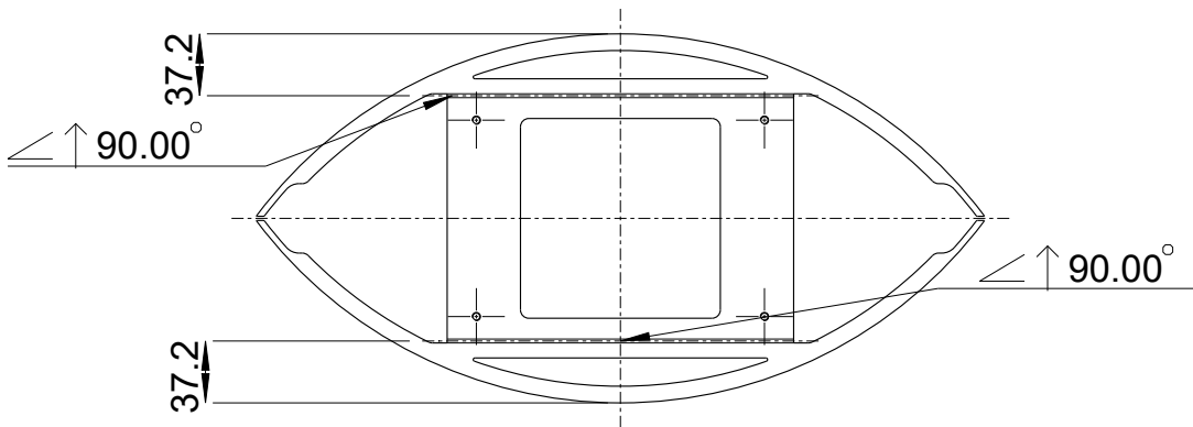
Zuschnitt laser contour 1:5
