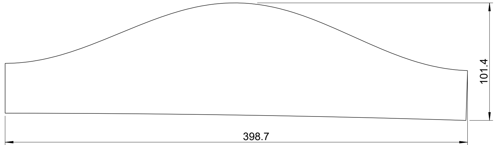
Zuschnitt 1:2
