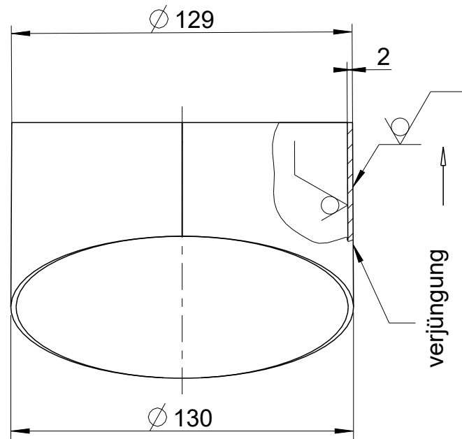
A-A
