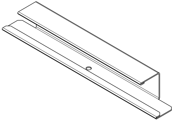
3D-Ansicht 1:2
