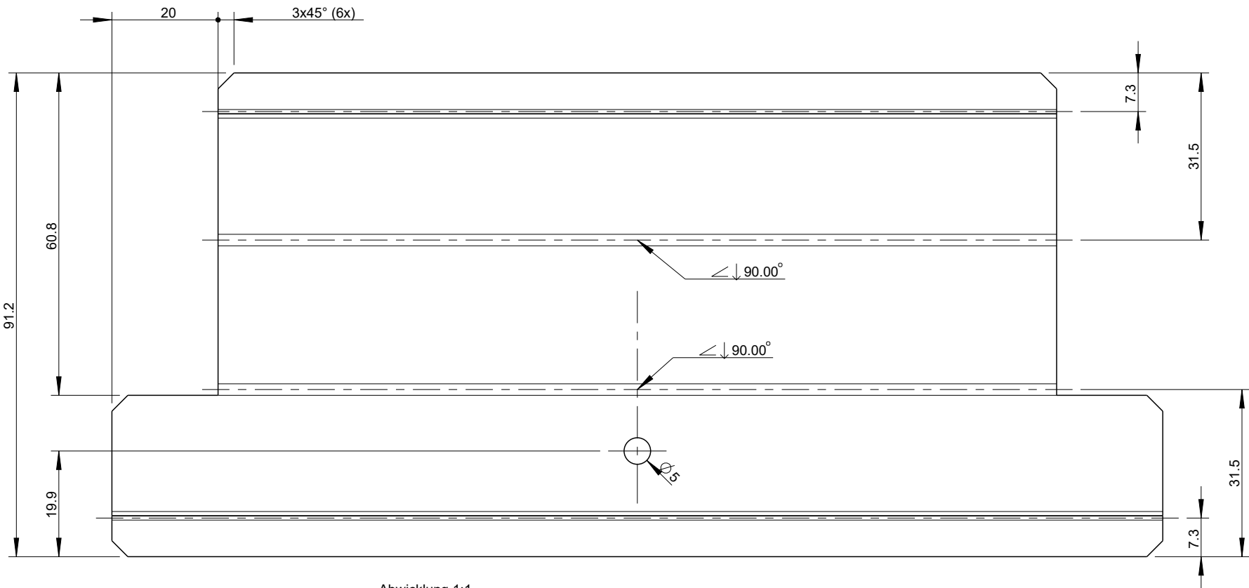
Abwicklung 1:1
