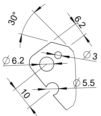
Detail Y 1:1
