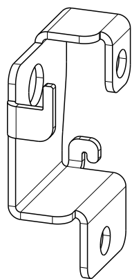
3D-Ansicht 1:1
